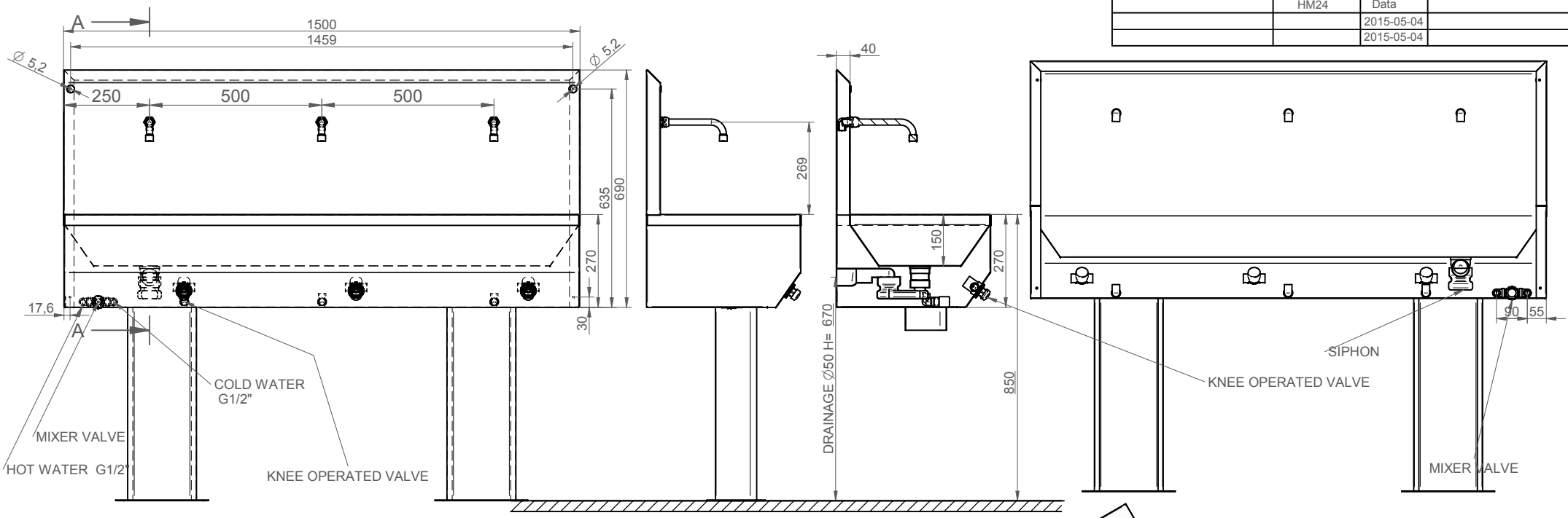
SECTION A-A
