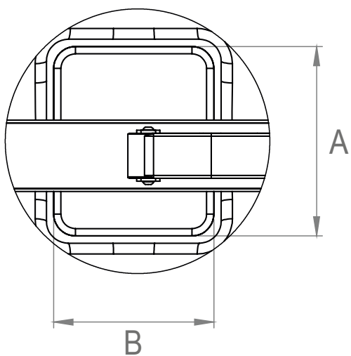
DETTAGLIO A
