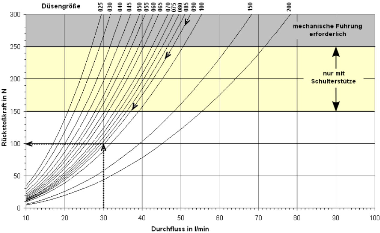
Diagramm zum Ermitteln der Haltekraft nach DIN EN 60335-2-79
